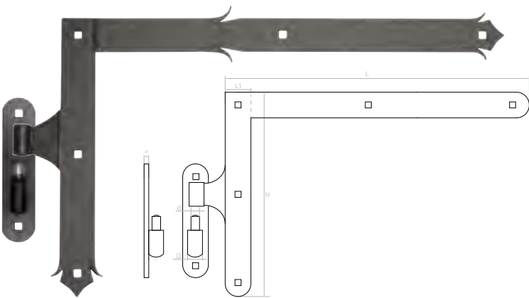
Zawias kątowy ozdobny Hinge / Петля / Scharnier
